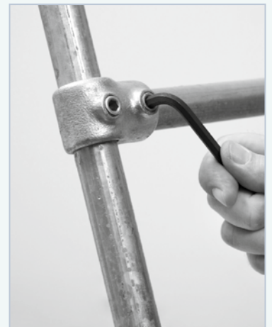
Montage met inbus
